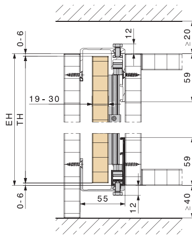
HAWA-Concepta 25/30 avec profil Connector 55 mm.
